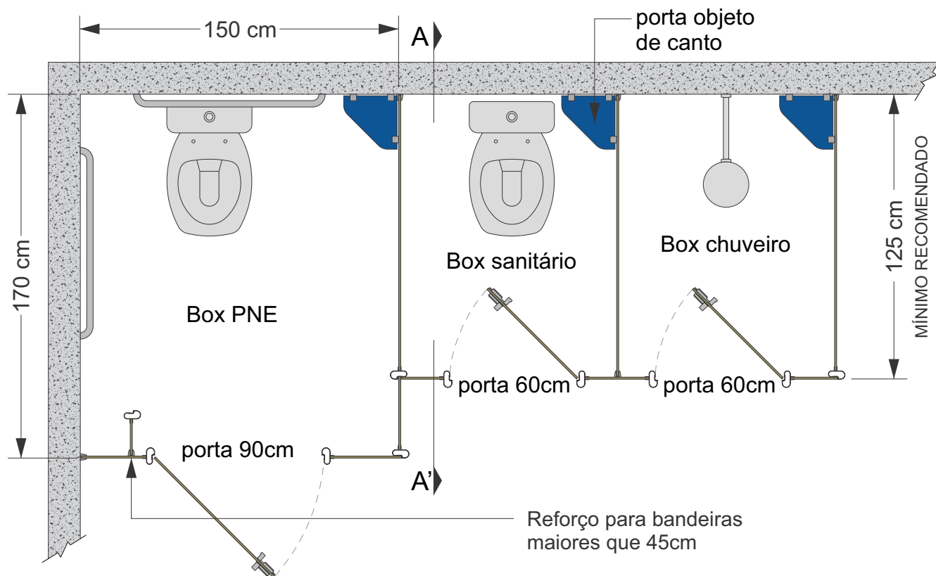
Planta baixa
