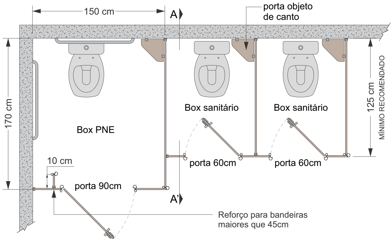
Planta baixa
