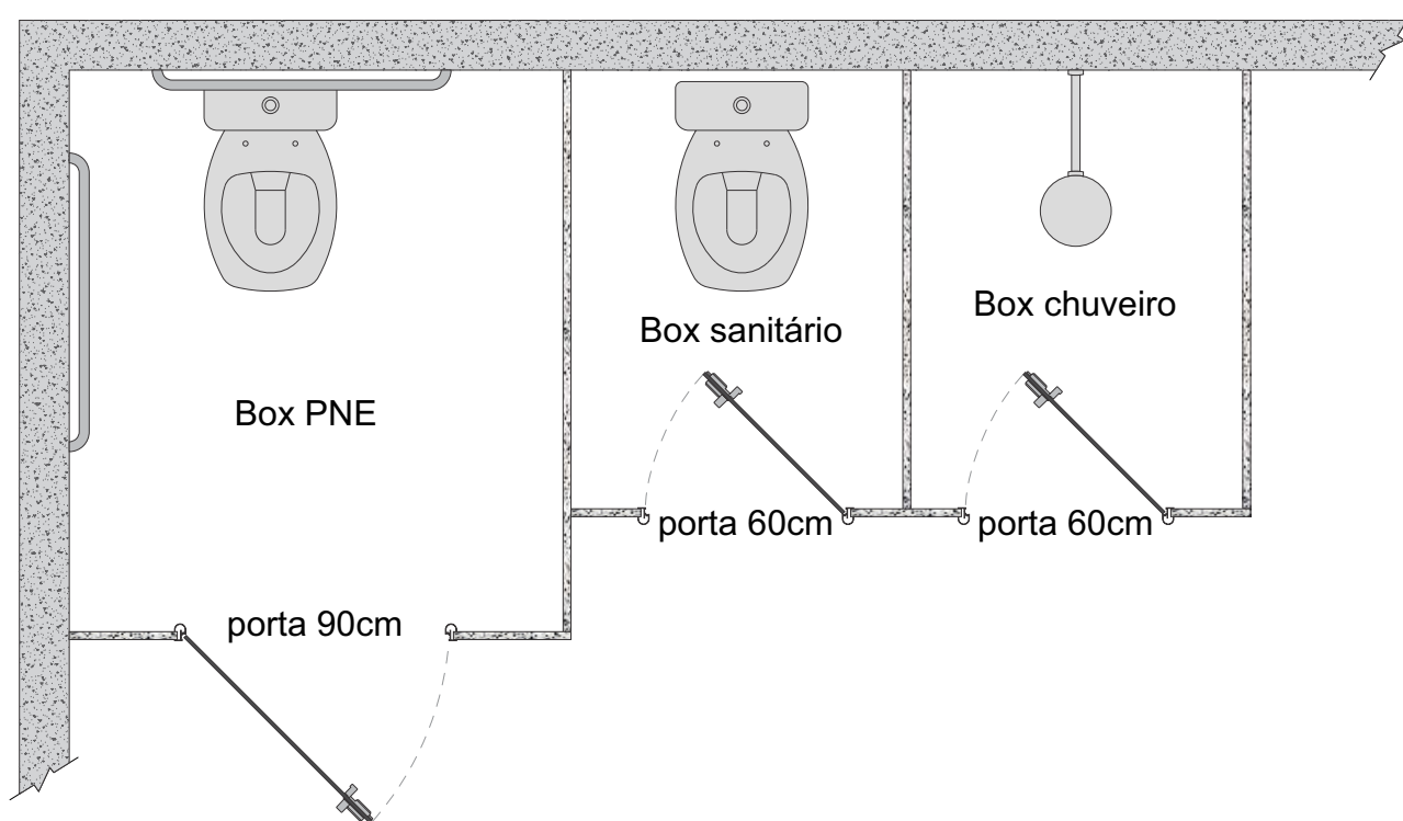
Planta baixa
